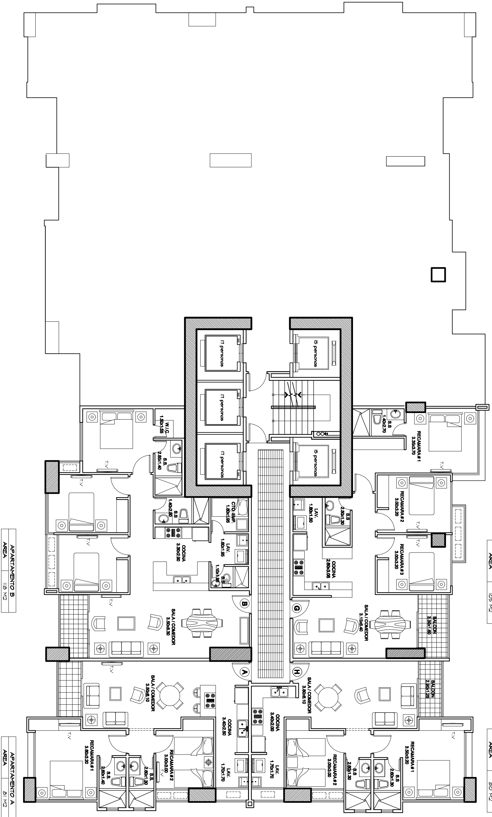
APARTAMENTO G AREA 105 M2
